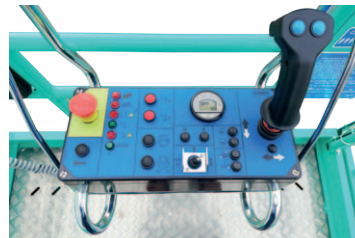
Einfacher und intuitiver Bedinpult, den man zum Laden / Entladen der Maschine aus der Plattform schnell runter nehmen kann
